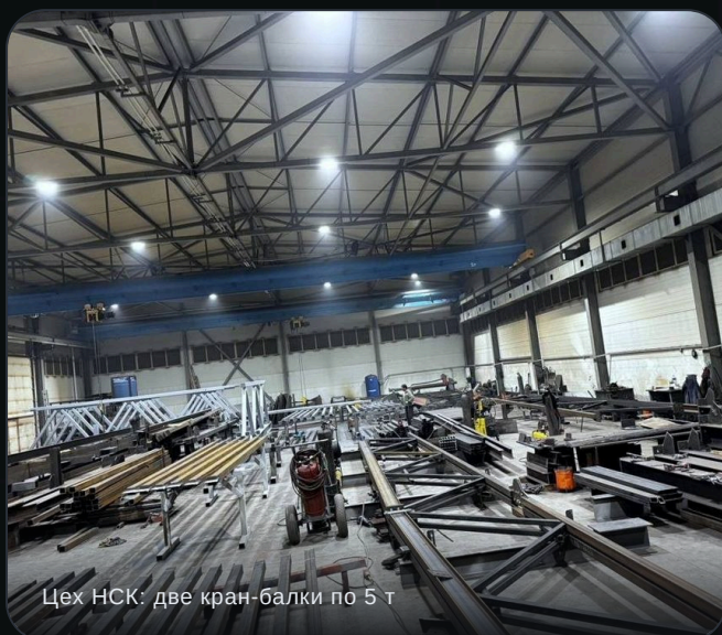
Сборка марок на сборочной плите
